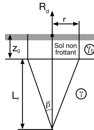
Figure G.5 : volume unitaire associé (sol frottant surmonté d'un sol sans frottement)
