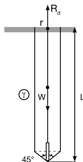
Figure G.2 : volume unitaire associé (sol cohérent)
