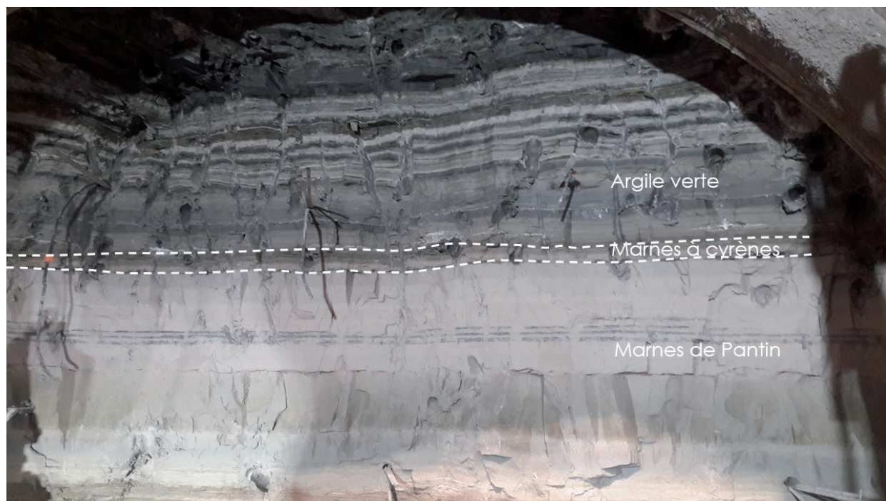
Front creusé dans les Argiles vertes de Romainville ici très litées et les Marnes « blanches » de Pantin. GPE, L14 Sud (Gare IGR = Villejuif-Gustave Roussy (anciennement Institut Gustave-Roussy)). Photographie F. Binet
