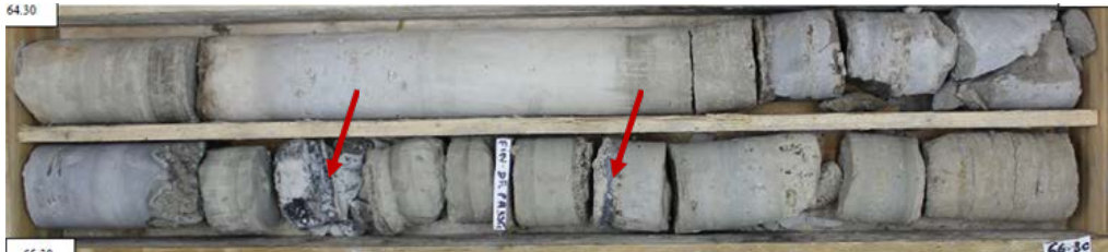
L15E_FSB-AVP-SC04302_Calcaire à intercalations fines de silex sombre (flèches rouges). Tiers supérieur de la formation (Calcaire grossier "supérieur")
