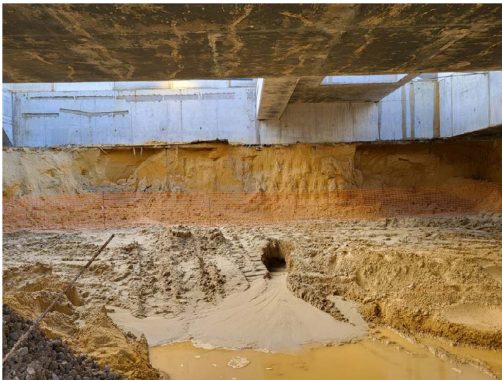
Excavation dans les Sables de Fontainebleau très altérés sur la ligne 18-3 à Versailles-Chantiers du GPE (Grand Paris Express). Photographie F. Binet
