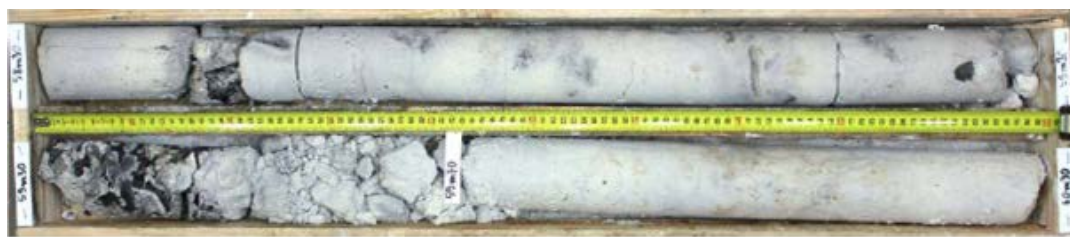
L15S_CHA-AVP-SC2337. Craie globalement massive à niveaux de silex noirs
