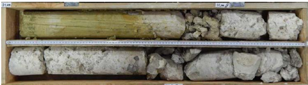
L16_CSM-PRO-SC332_Calcaire tendre vert kaki et calcaire franc, dur et vacuolaire
