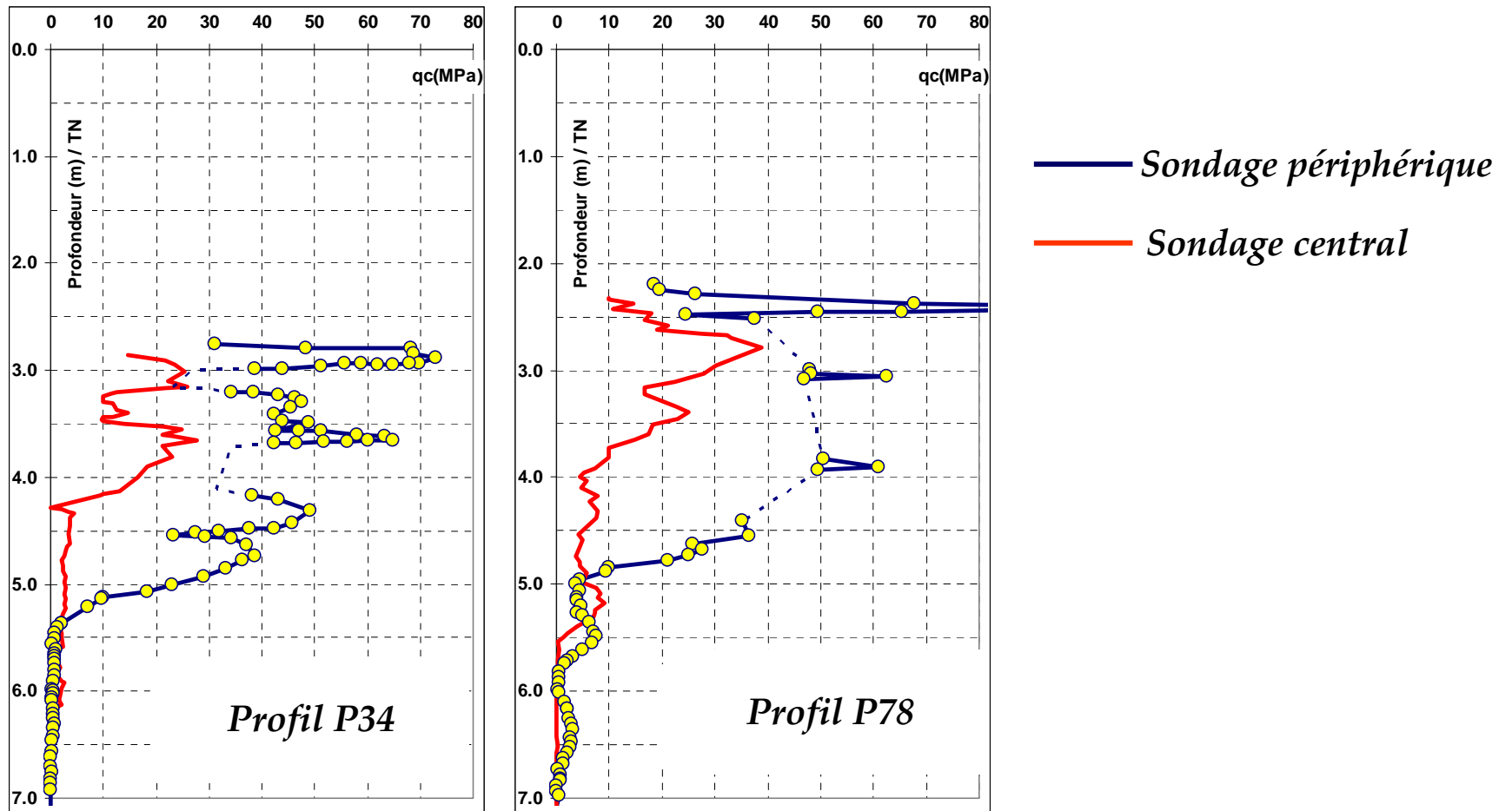
Profils en travers en zone de résurgences
