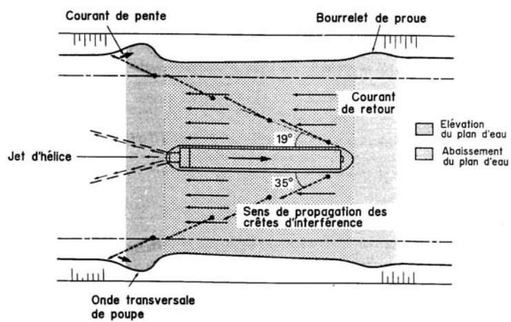
FIG. 3.9 : Composantes de l'agitation de l'eau induite par la navigation
