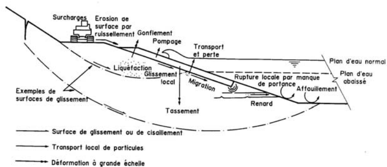
FIG. 3.13 : Mécanismes de rupture du sous-sol
