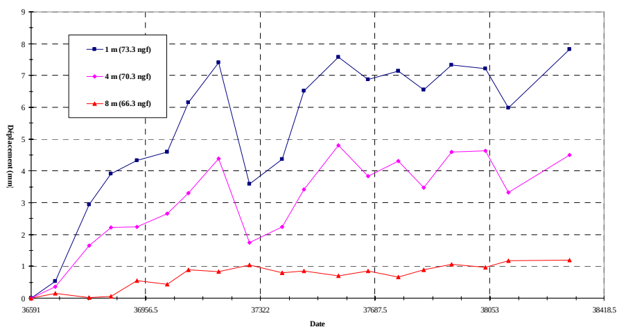
Grand Littoral Inclinomètre IPA24 - Talus Barnier Résultante des composantes AA et BB
