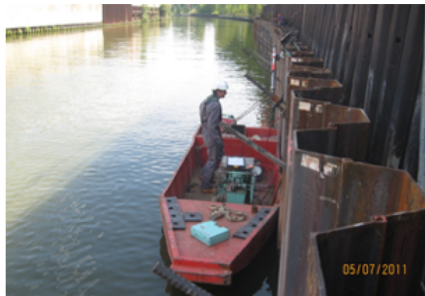
Photo 7.17 : Exemple de mise en tension de tirants sur un rideau de palplanches
