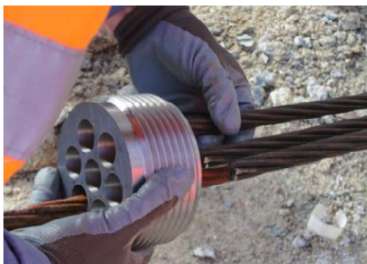
Photo 3.4b : Bloc d'ancrage retensionnable (© Freyssinet)
