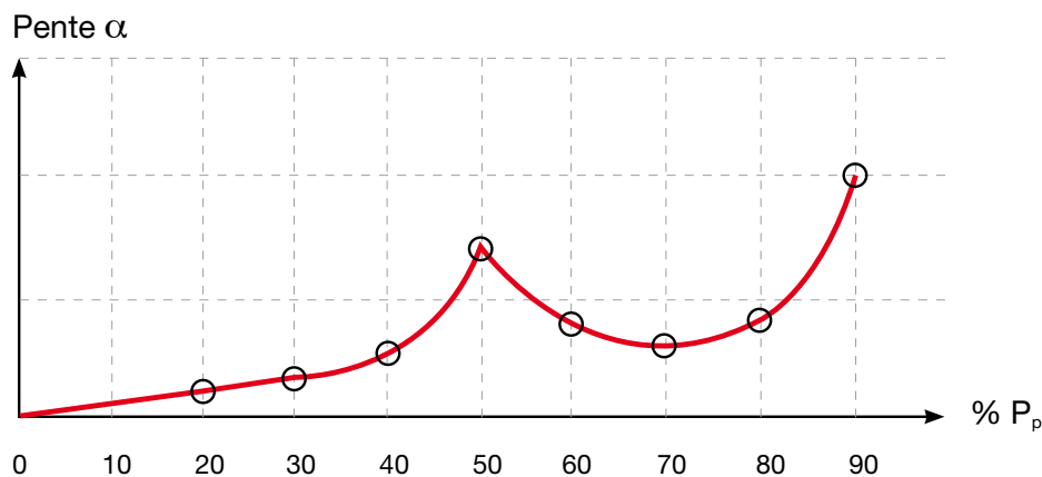
Figure 8.3 : exemple d'un essai comportant une anomalie
