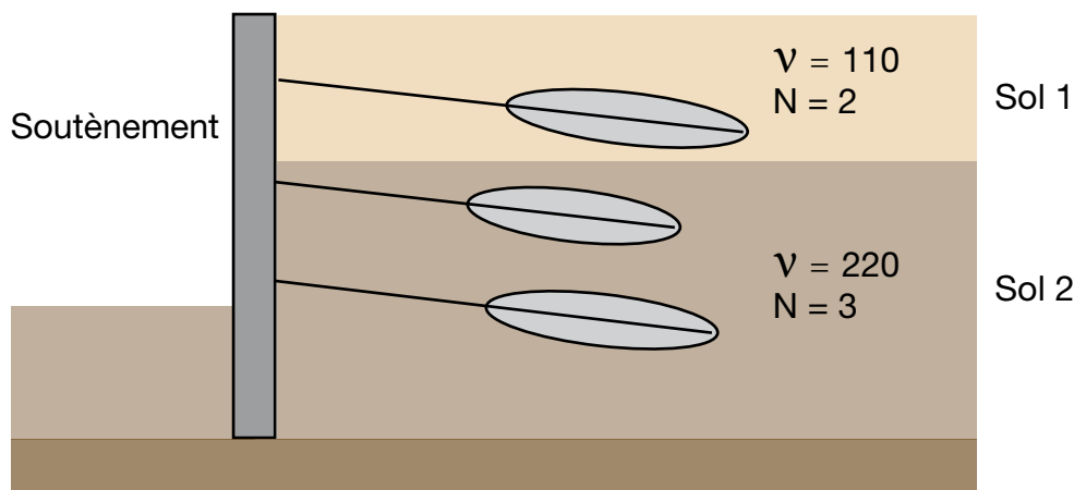
Figure 8.2 : exemple d'un sol bicouche
