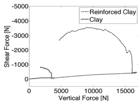
Figure 5. Swipe test pour le sol argileux non renforcé et le sol renforcé avec Colonnes Mixtes.
