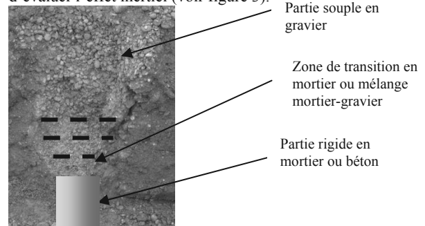
Figure 1. Dégarnissage d'une Colonne Mixte, Niederbipp (CH).
