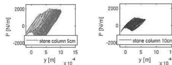
Figure 8. Courbes p-y en tête de la partie rigide pour 5 et 10 cm de colonne de gravier.
