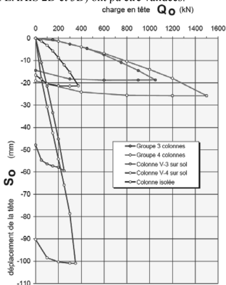
Figure 2. résultats des essais sur sol vierge (courbes bleues) et du sol renforcé par Colonnes Mixtes (courbes rouges).
