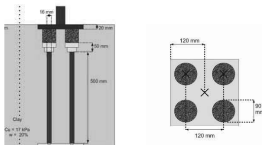
Figure 3. Modèle mixte échelle 1/10 (Thèse Hana Santruckova 2012).
