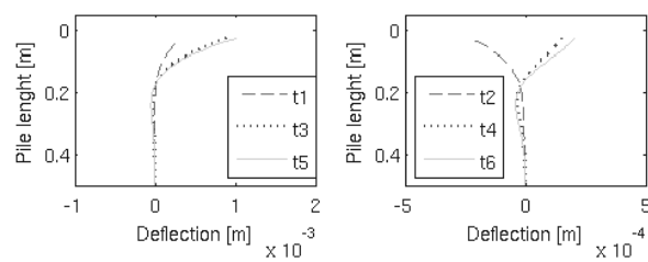
Figure 6. Profils de déplacements pour les temps t1 à t6 (hauteur partie souple 5 cm).
